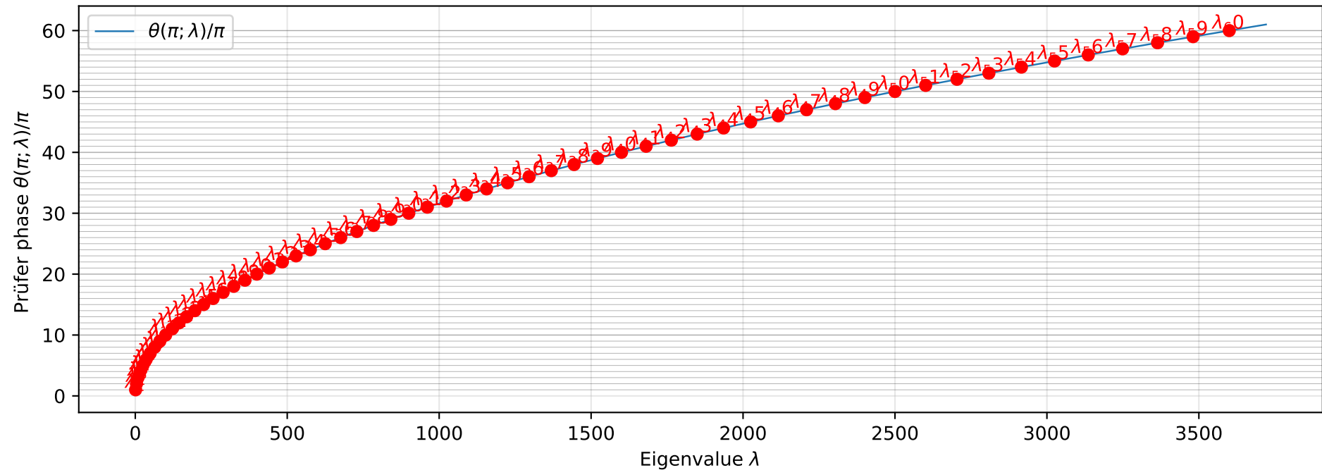
Prüfer phase sweep on uniform grid (n=100) for 60 eigenvalues
